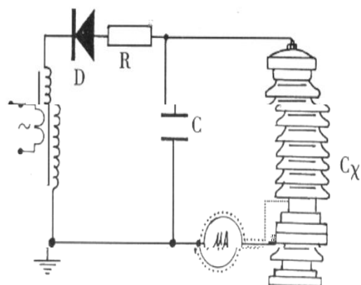
2. 排除试品 C_X 表面影响接线图
