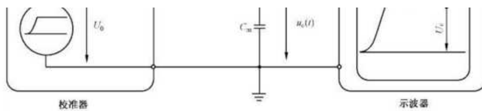
图 B.3 采用阶跃电压法对校准器进行性能试验的回路图
