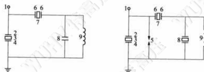
a) 内部无放电间隙的放电记录器
