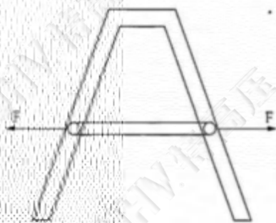
图C.14 人字梯网张装置强度试验示意图
